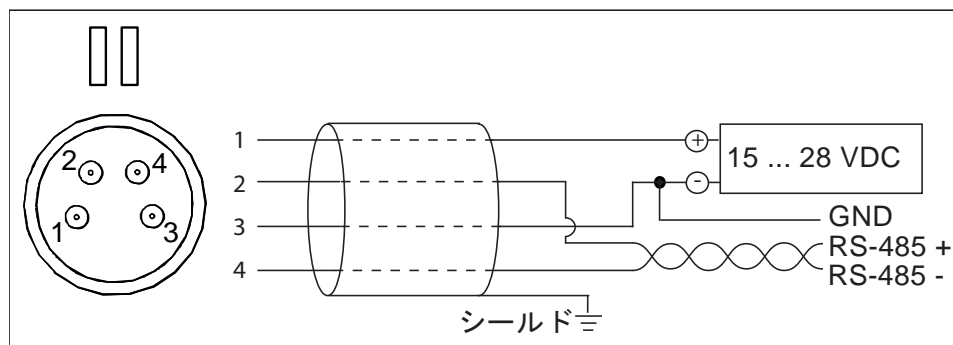
ヴァイサラケーブルの配線色
